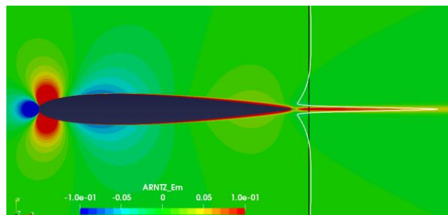
Figure 3 : Distribution d'exergie mécanique NACA 0012, M=0.3 [4]
