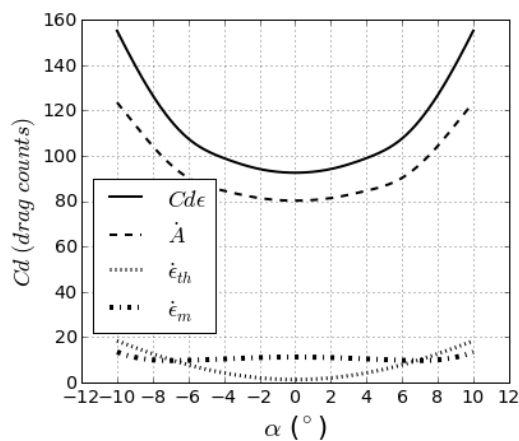
Figure 2 : Décomposition de traînée par analyse exergétique [3]
